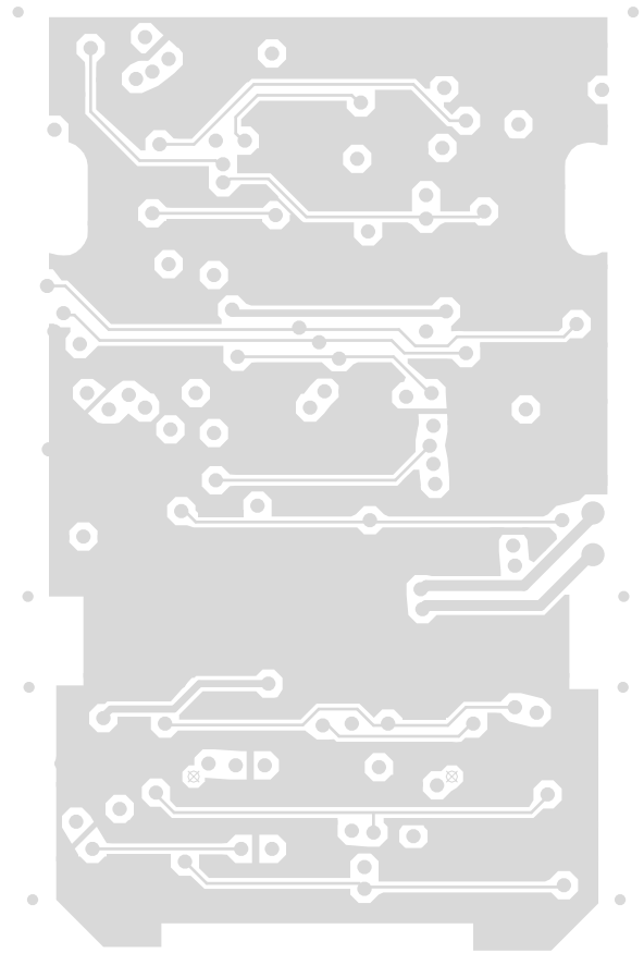
ORCA KEYPAD INTERFACE 220-01412-00 A LAYER 2
