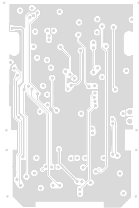
ORCA KEYPAD INTERFACE 220-01412-00 A LAYER 3
